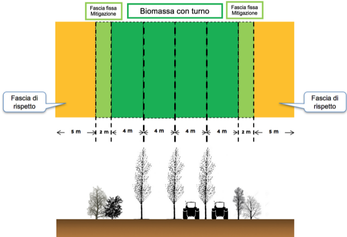
Fig.2 - Struttura funzionale delle fasce boscate di mitigazione con produzione di biomassa
