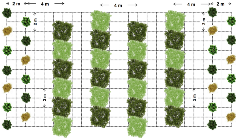
Fig. 1 - Modulo di impianto tipo
